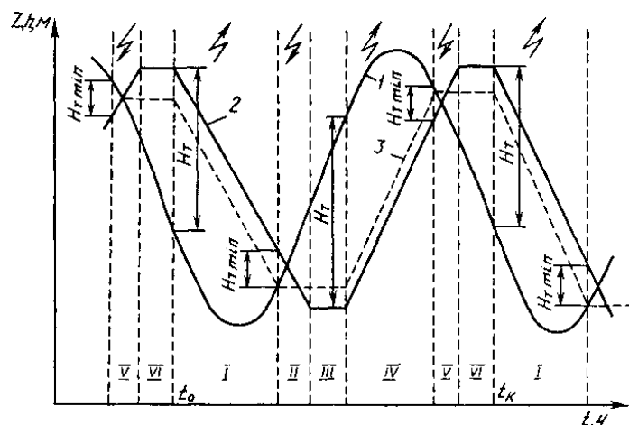
Рис.4. Схема работы одnobассейновой ПЭС двустороннего действия.
