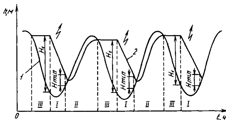
Рис.3. Схема работы односторонней ПЭС одностороннего действия:
