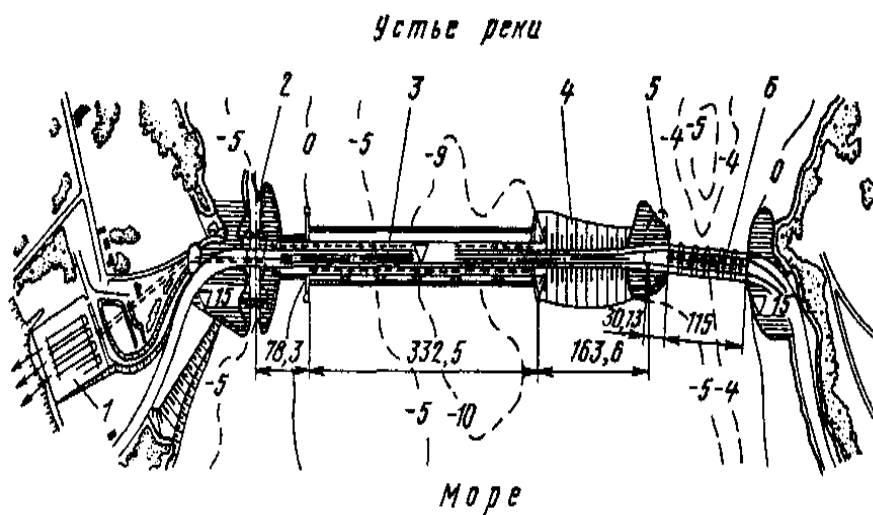
Рис.5. План сооружений ПЭС Ране:
