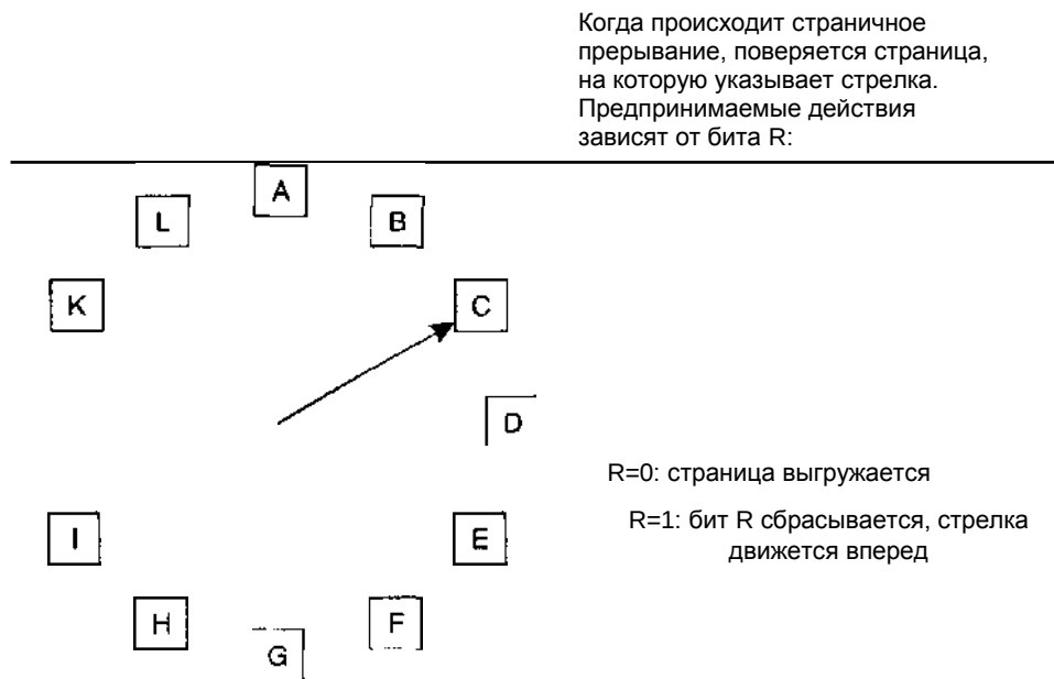
Рис. 6. Алгоритм замещения страниц «часы»
