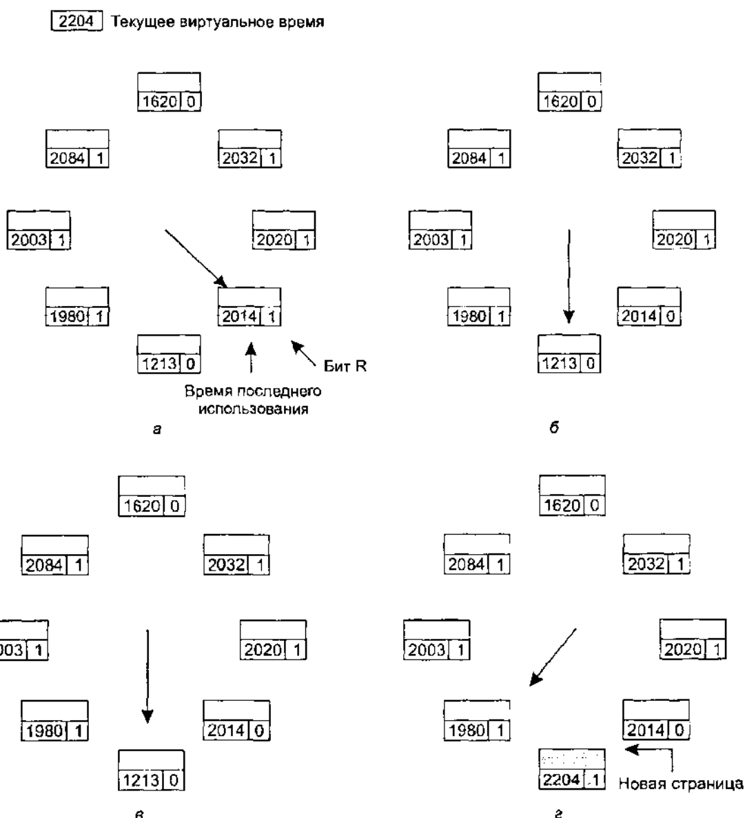
Рис. 10. Работа алгоритма WSClock: пример того, что происходит при бите R = 1 (а) и (б); пример для бита R = 0 (в) и (г)
