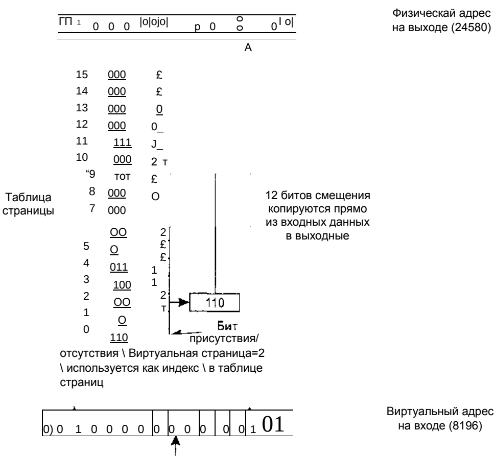
Рис. 1. Внутренняя операция MMU в системе с шестнадцатью страницами размером 4 Кбайт
