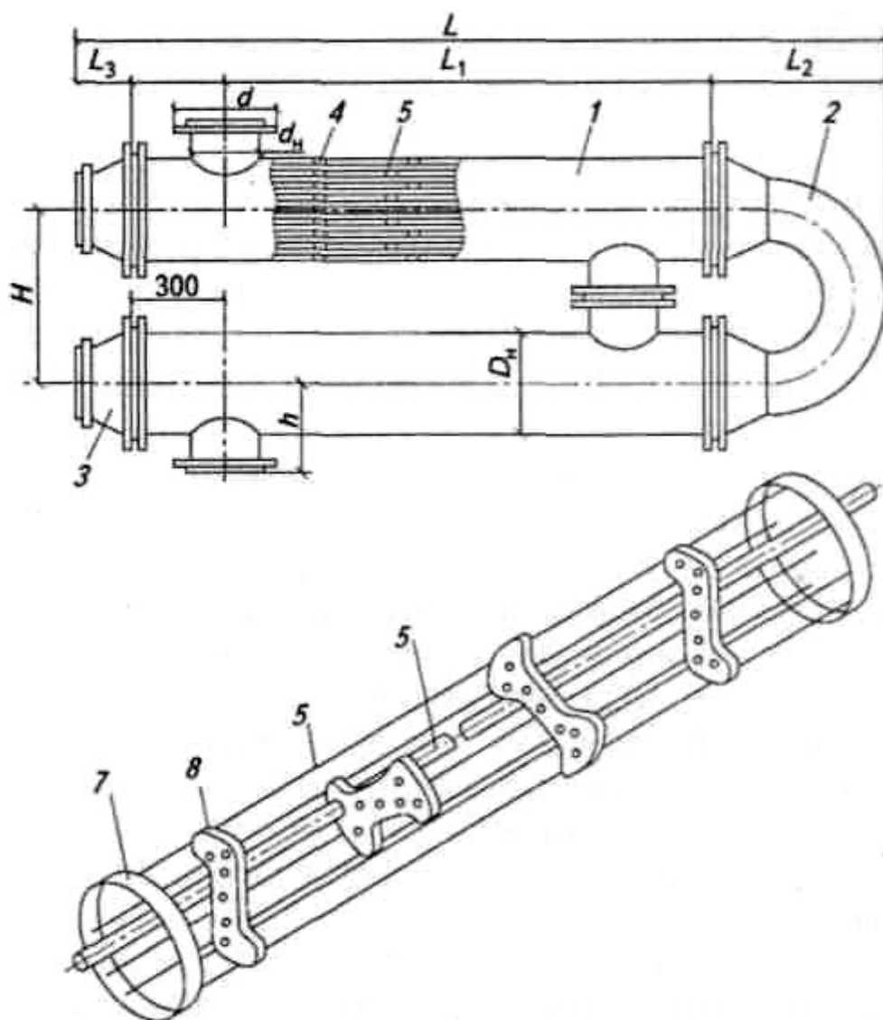
Рис. 46. Общий вид горизонтального секционного кожухотрубного водоподогревателя (ВВП) с опорами-турбулизаторами по ГОСТ 27590 1 - секция ВВП; 2 - калач; 3 - переход; 4 - блок опорных перегородок; 5 - трубки; 6 - перегородка опорная; 7 - кольцо; 8 – пруток
