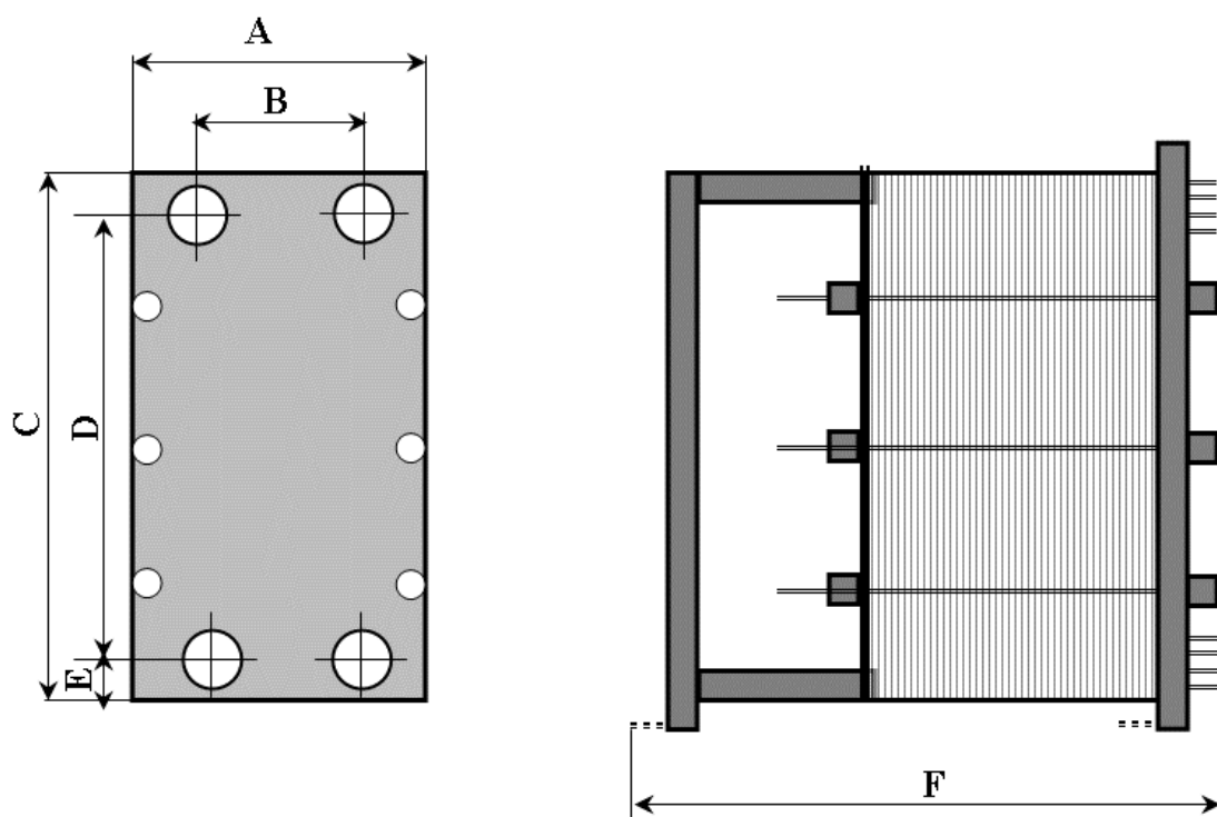
Рис. 47. Принципиальная схема разборного пластинчатого теплообменника «Alfa Laval»
