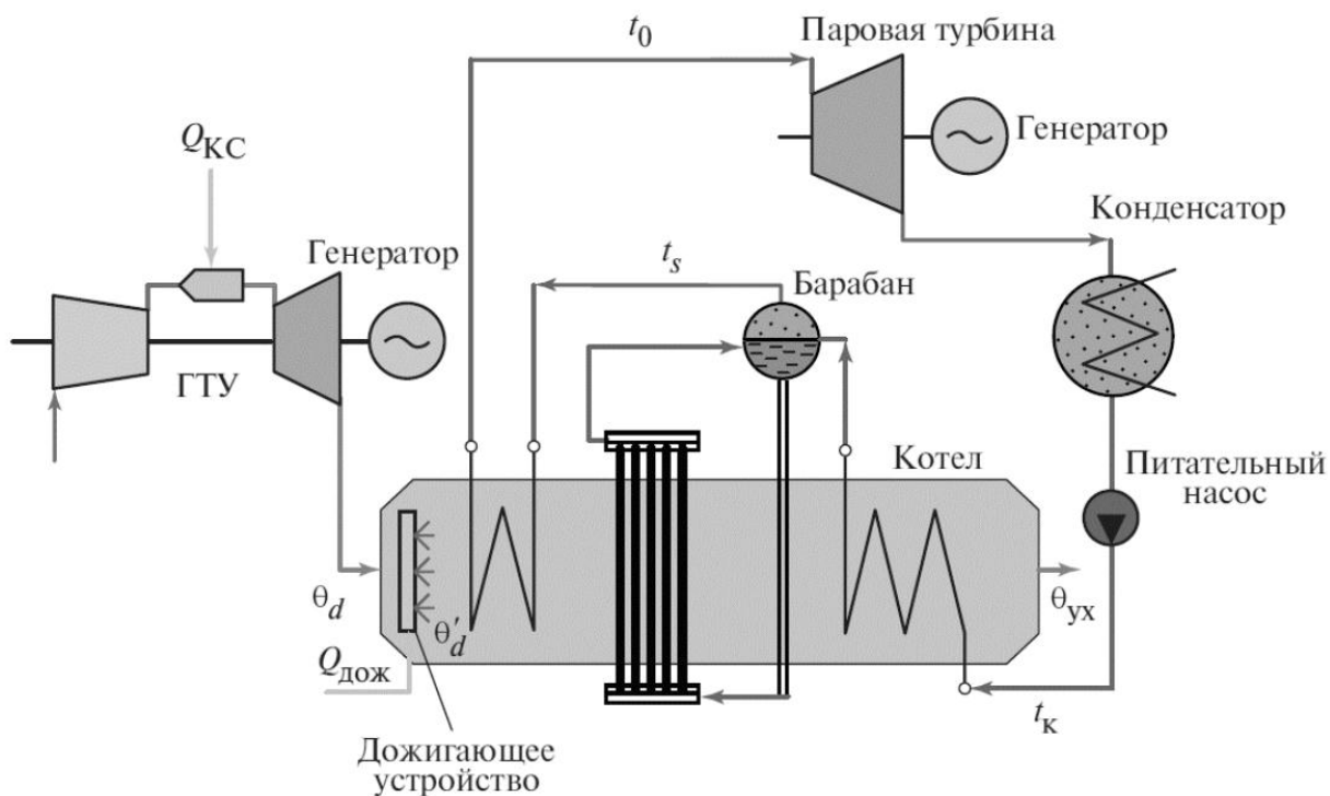
Рис. 2.16. Схема простейшей ПГУ с дожиганием.
