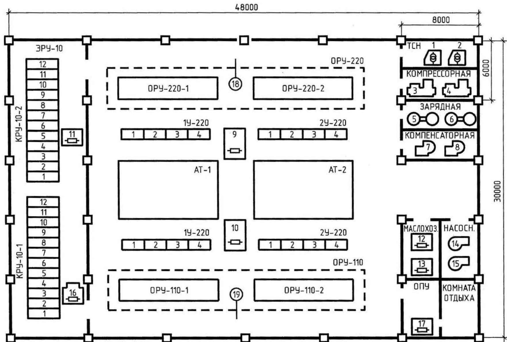
Рис. 3.20. План расположения ЭО узловой распределительной подстанции
