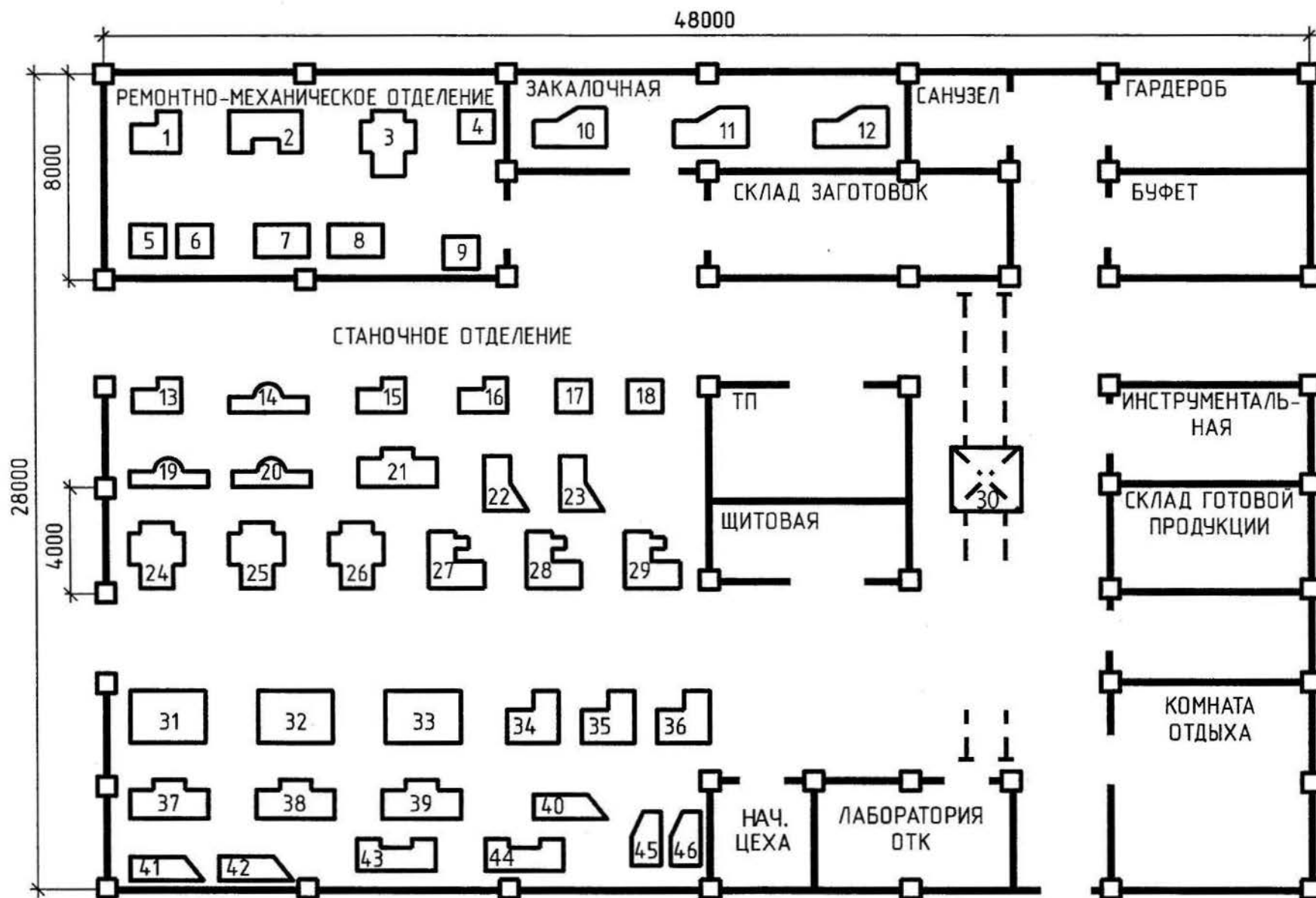
Рис. 3.10. План расположения ЭО цеха механической обработки деталей
