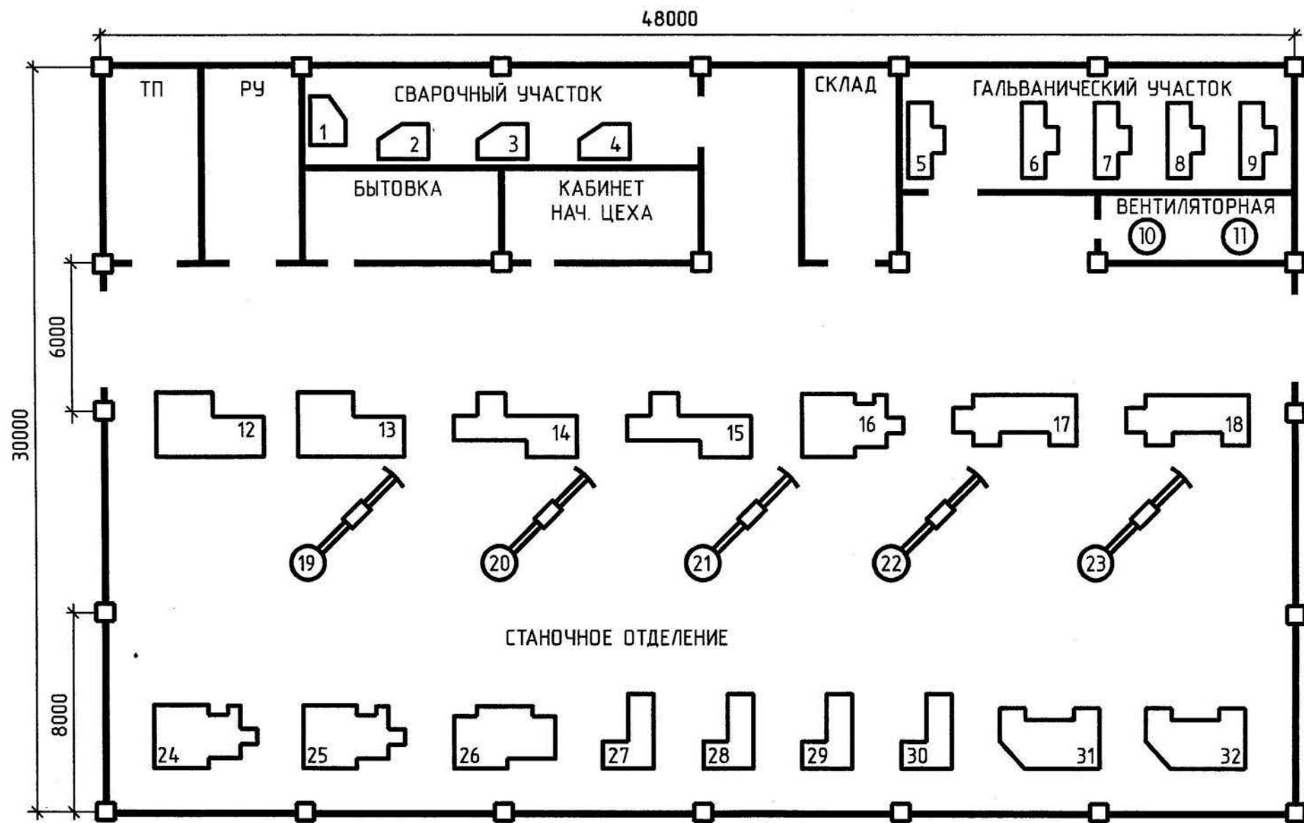
Рис. 3.6. План расположения ЭО цеха обработки корпусных деталей
