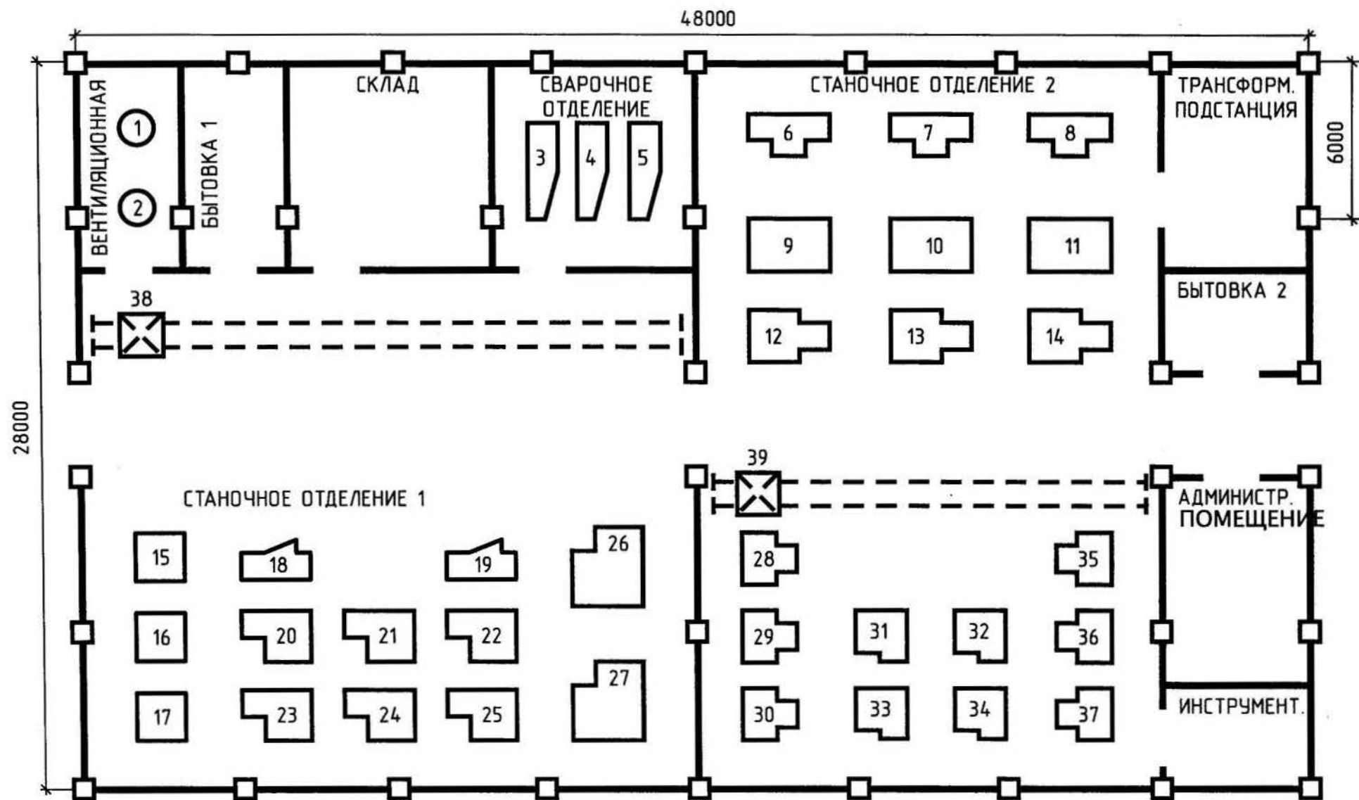
Рис. 3.1. План расположения ЭО ремонтно-механического цеха
