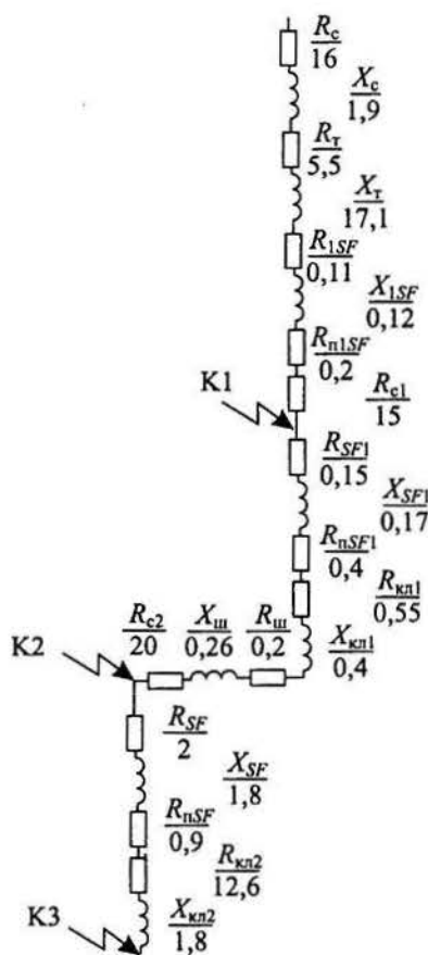
Рис. 1.9.3. Схема замещения
