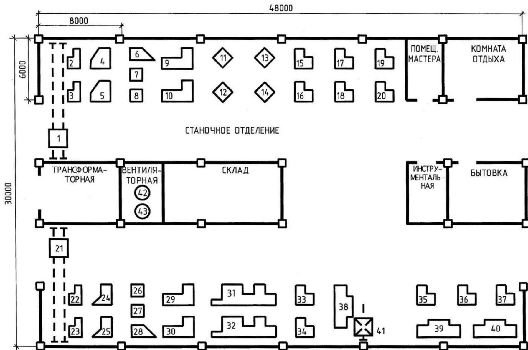
Рис. 3.3. План расположения ЭО электромеханического цеха
