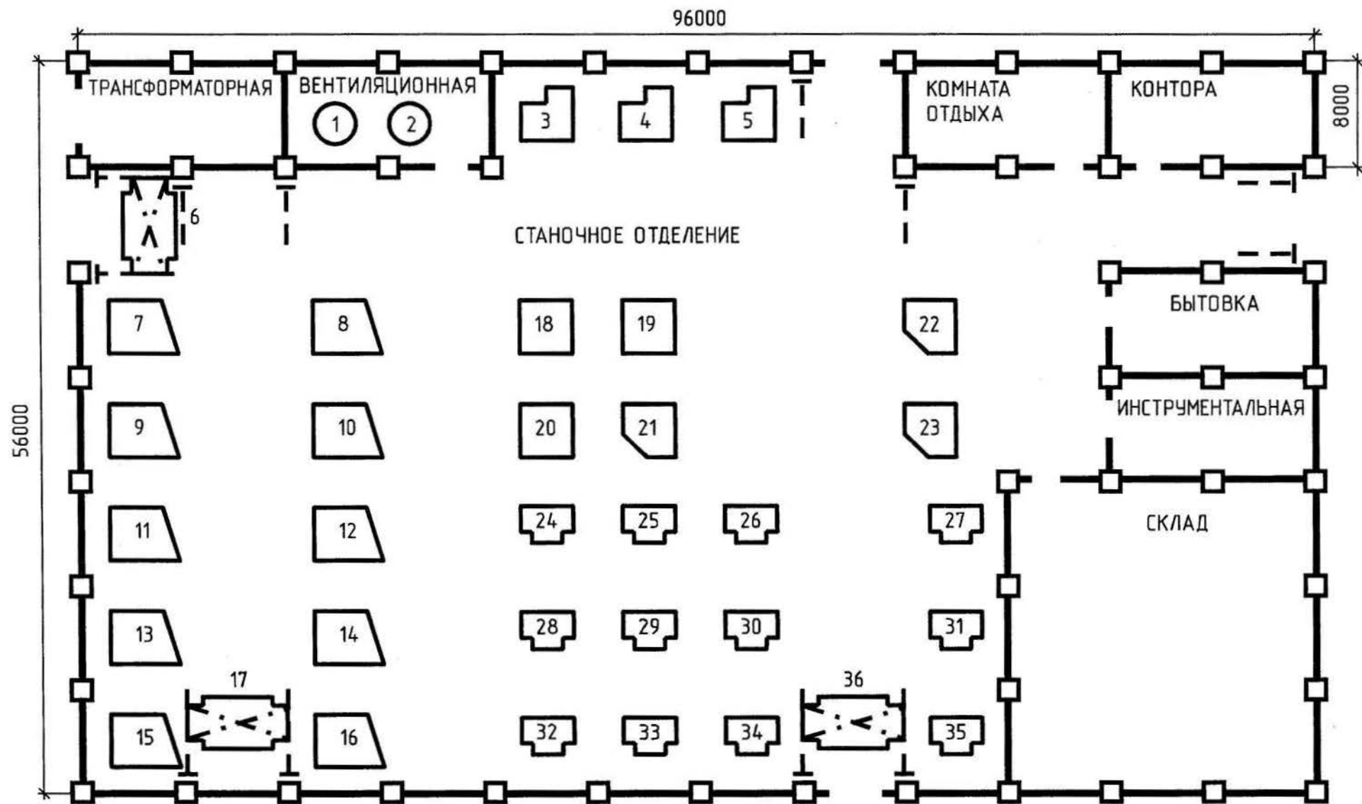
Рис. 3.2. План расположения ЭО участка кузнечно-прессового цеха
