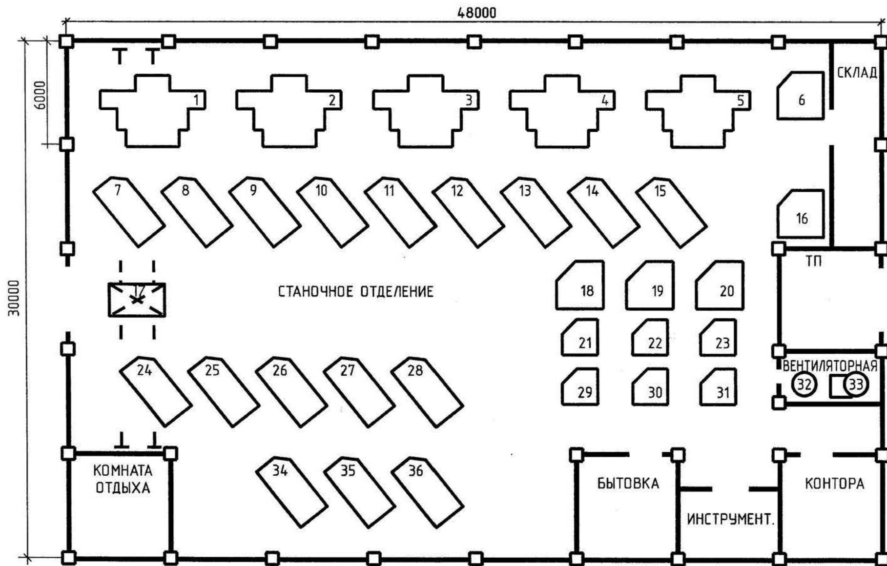
Рис. 3.5. План расположения ЭО механического цеха тяжелого машиностроения
