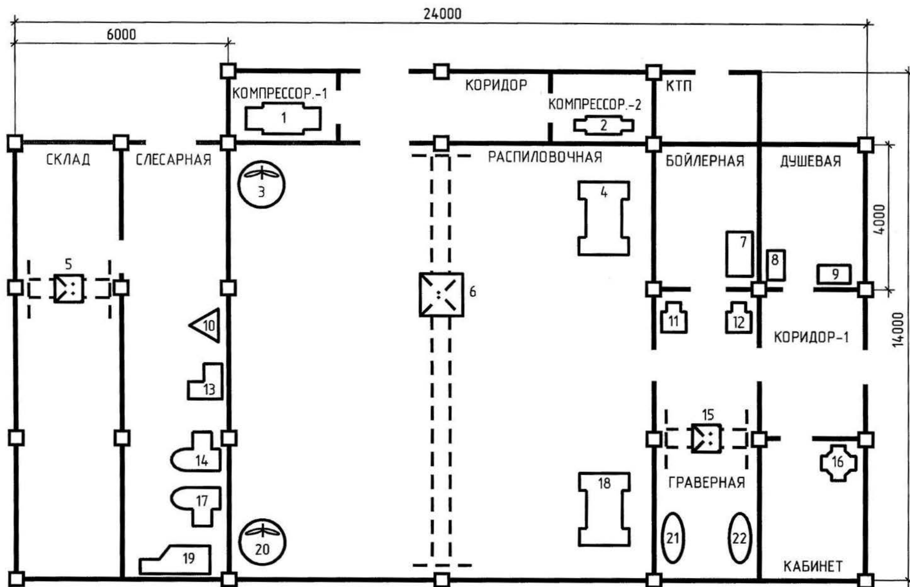
Рис. 3.22. План расположения ЭО гранитной мастерской
