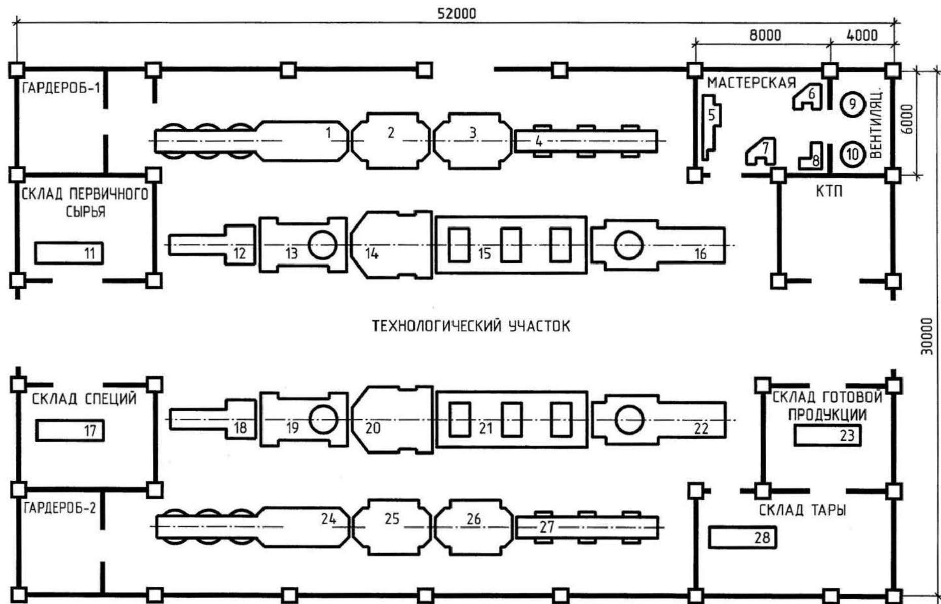
Рис. 3.21. План расположения ЭО комплекса томатного сока
