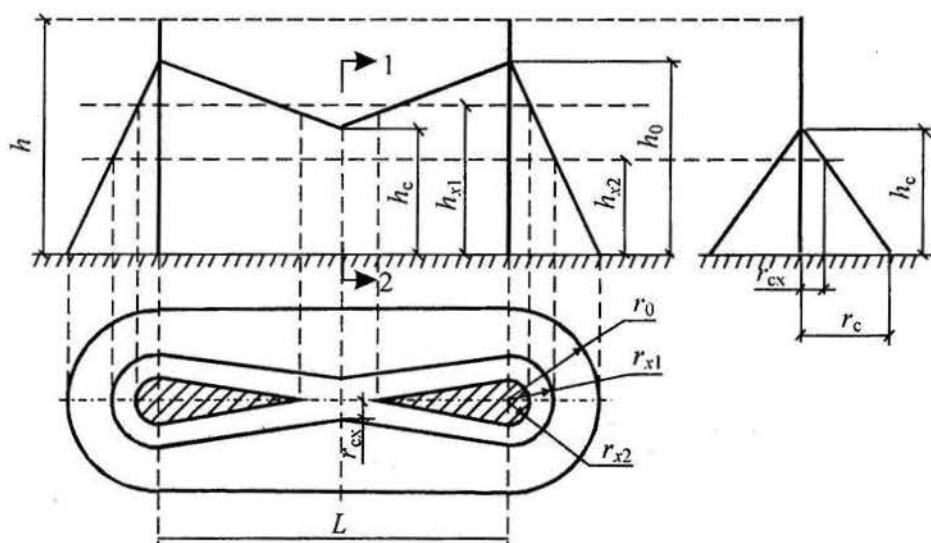
Рис. 1.14.2. Зона защиты двойного стержневого молниеотвода равной длины
