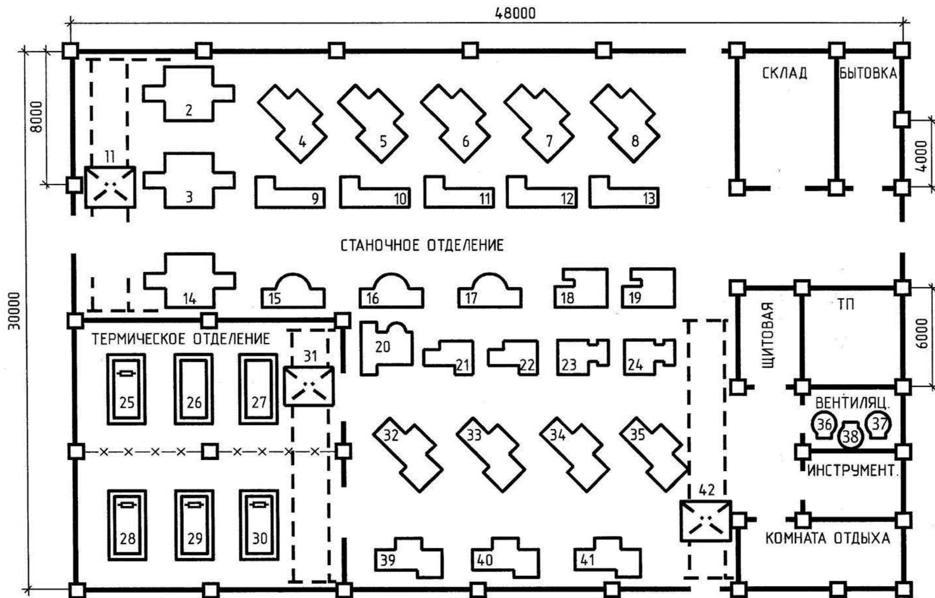
Рис. 3.13. План расположения ЭО цеха металлоизделий
