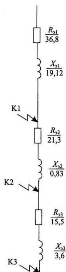
Рис. 1.9.4. Схема замещения упрощенная
