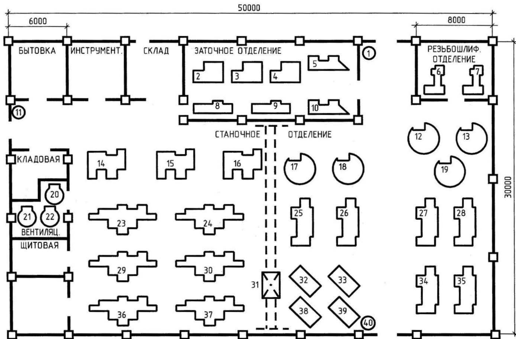
Рис. 3.15. План расположения ЭО цеха металлорежущих станков
