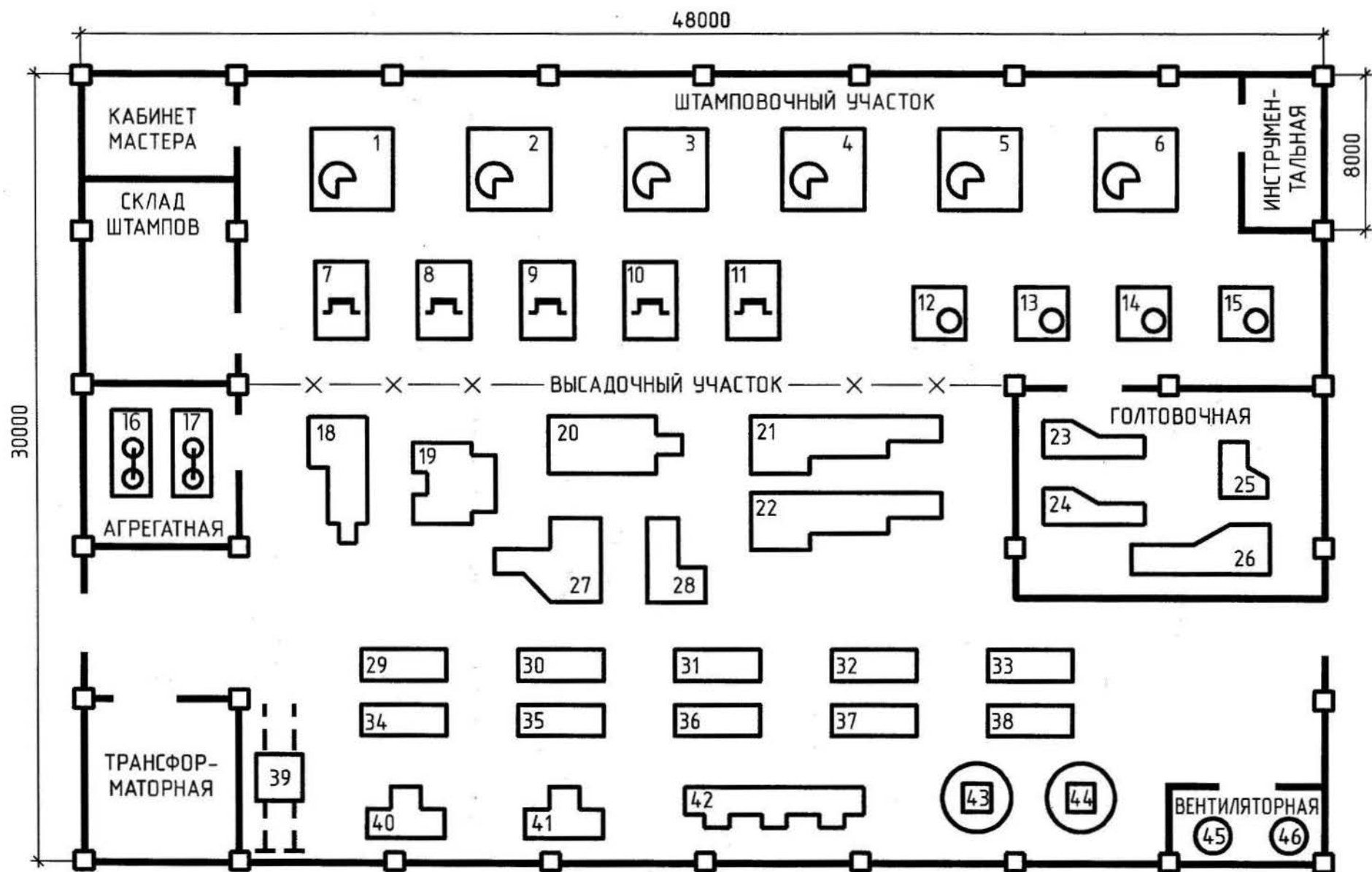
Рис. 3.4. План расположения ЭО автоматизированного цеха
