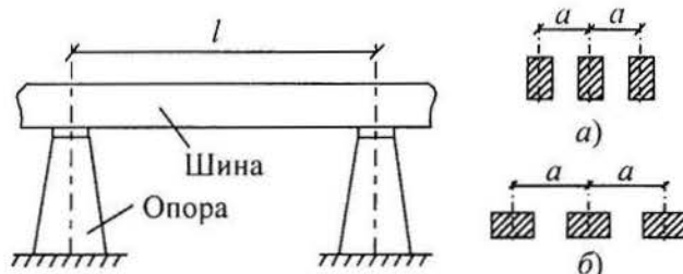
Рис. 1.10.1. Установка шин на опорах:
