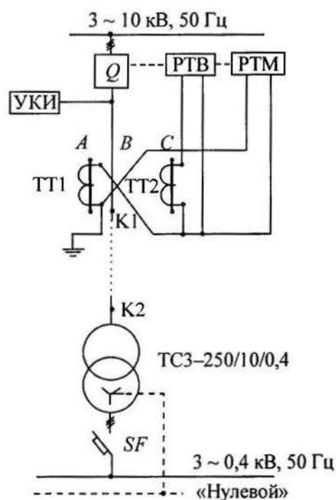
Рис. 1.12.2. Схема РЗ
