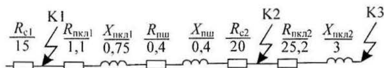
Рис. 1.9.5. Схема замещения для расчета 1-фазных токов КЗ
