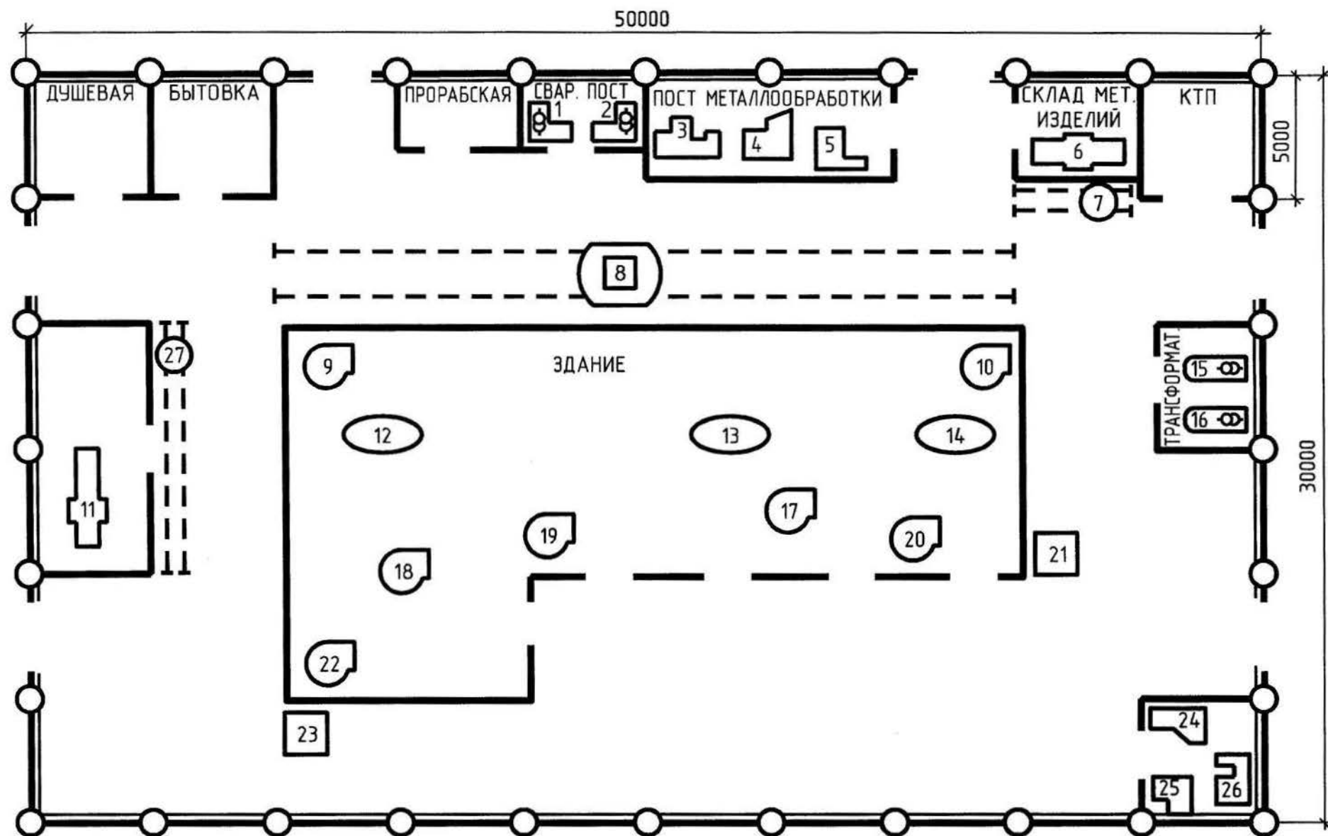
Рис. 3.19. План расположения ЭО строительной площадки жилого дома
