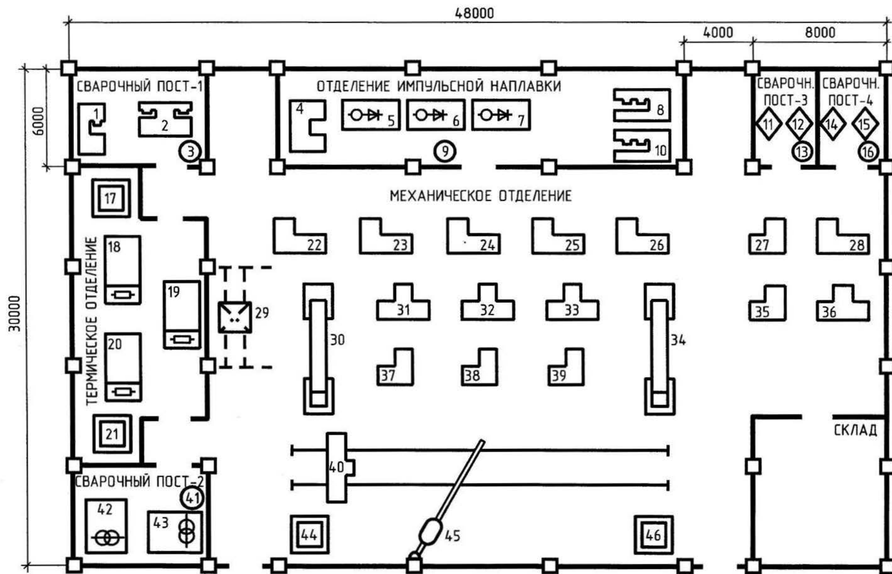
Рис. 3.16. План расположения ЭО сварочного участка цеха
