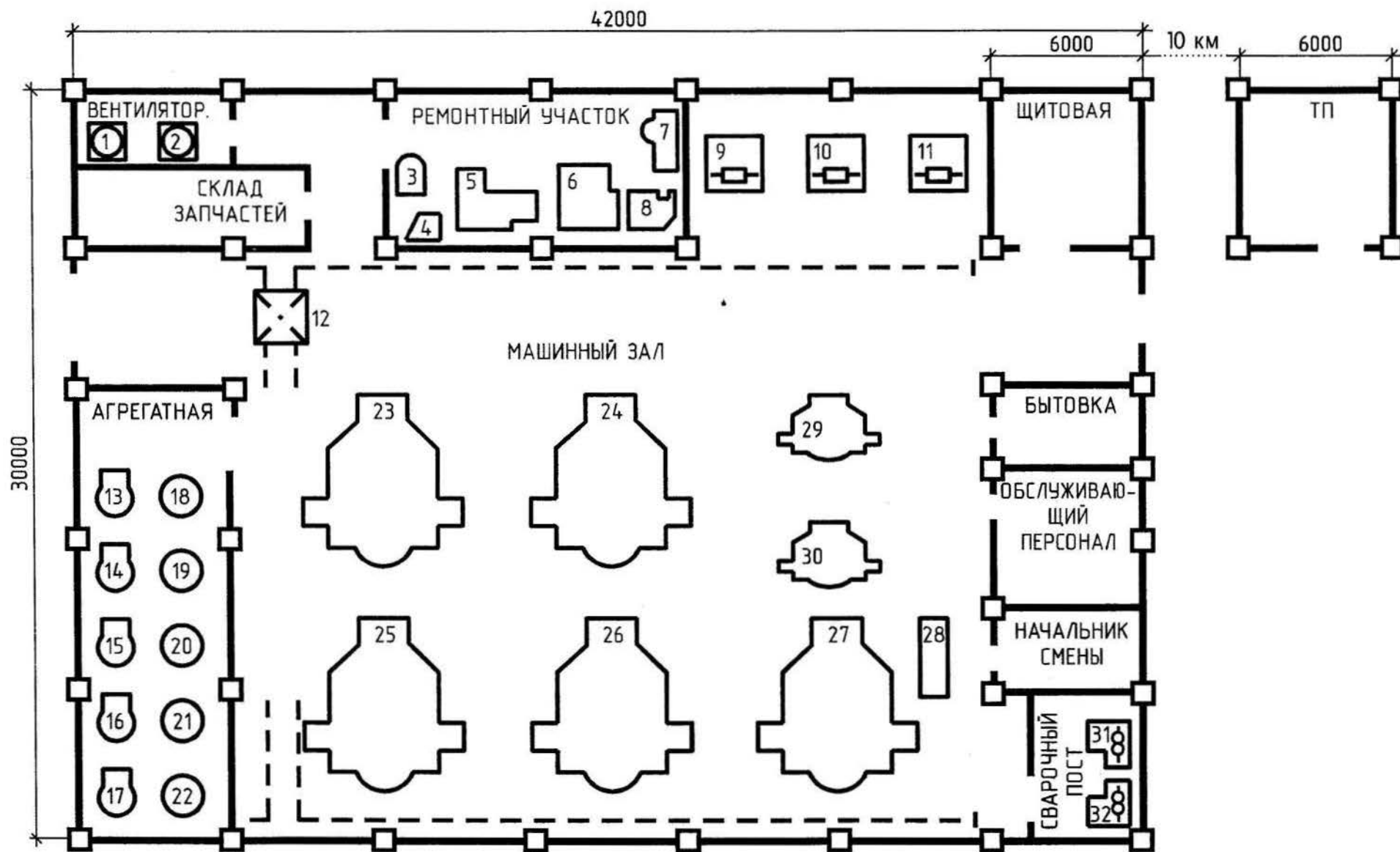
Рис. 3.8. План расположения ЭО насосной станции
