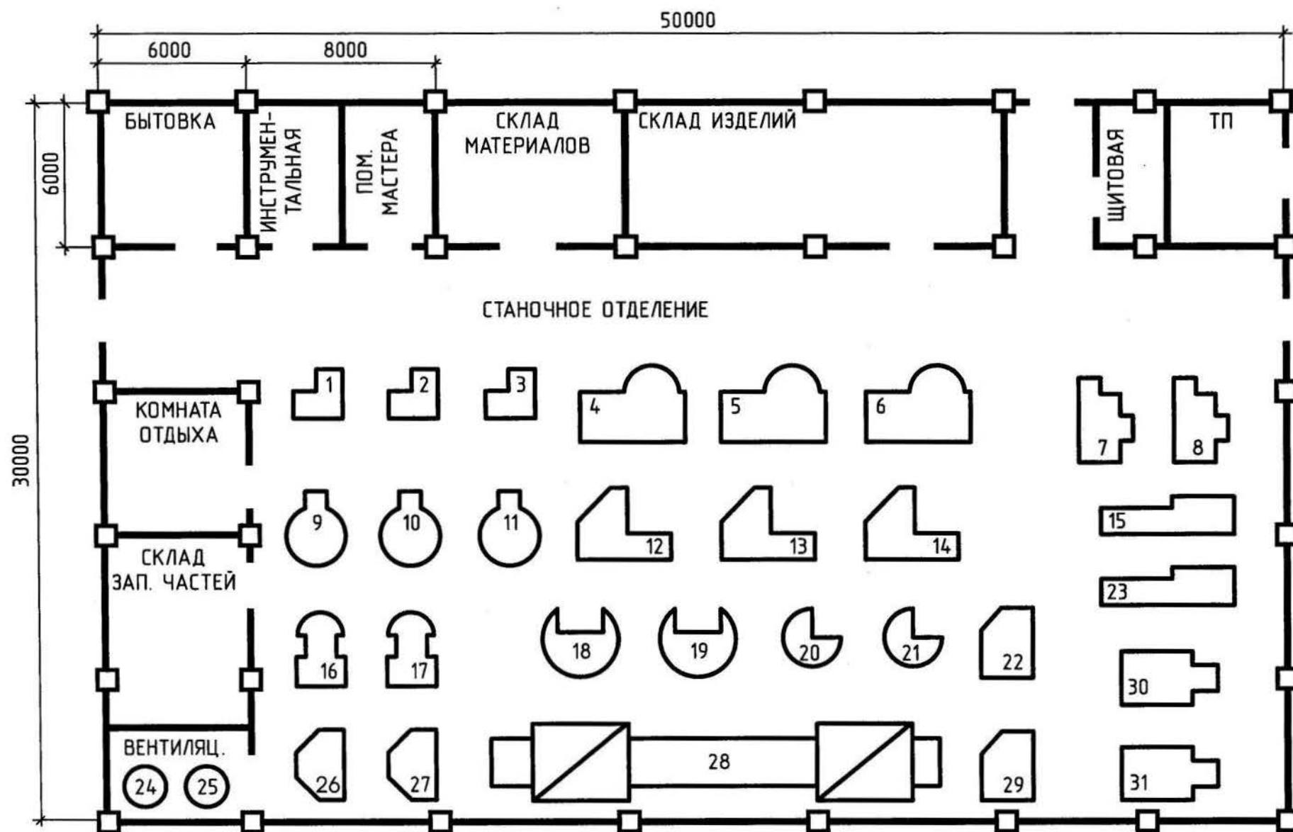
Рис. 3.14. План расположения ЭО участка механосборочного цеха
