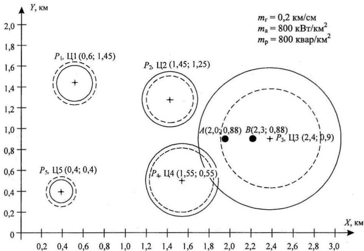
Рис. 1.7.1. Картограмма нагрузок
