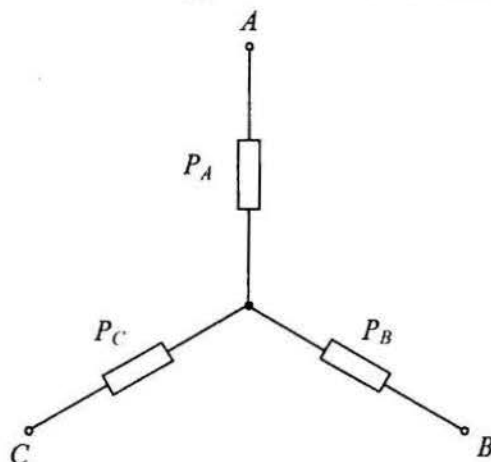
Рис. 1.5.2. Схема включения 1-фазных нагрузок на фазное напряжение
