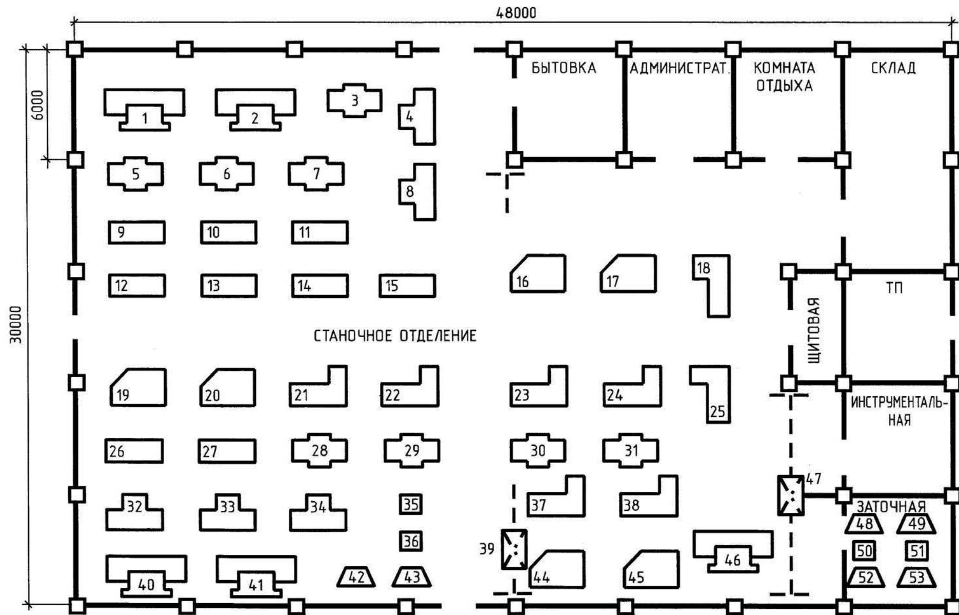
Рис. 3.11. План расположения ЭО инструментального цеха
