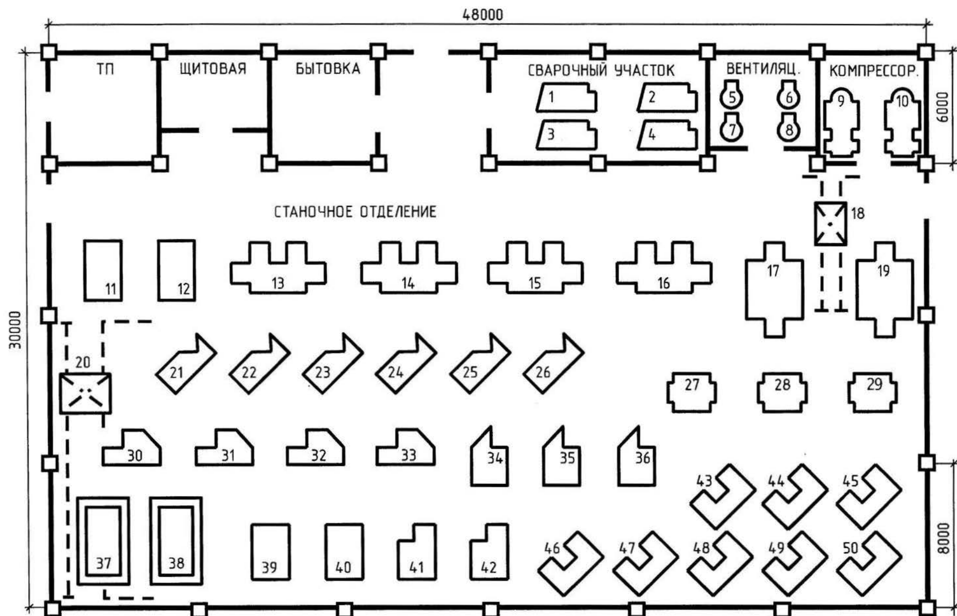
Рис. 3.12. План расположения ЭО механического цеха
