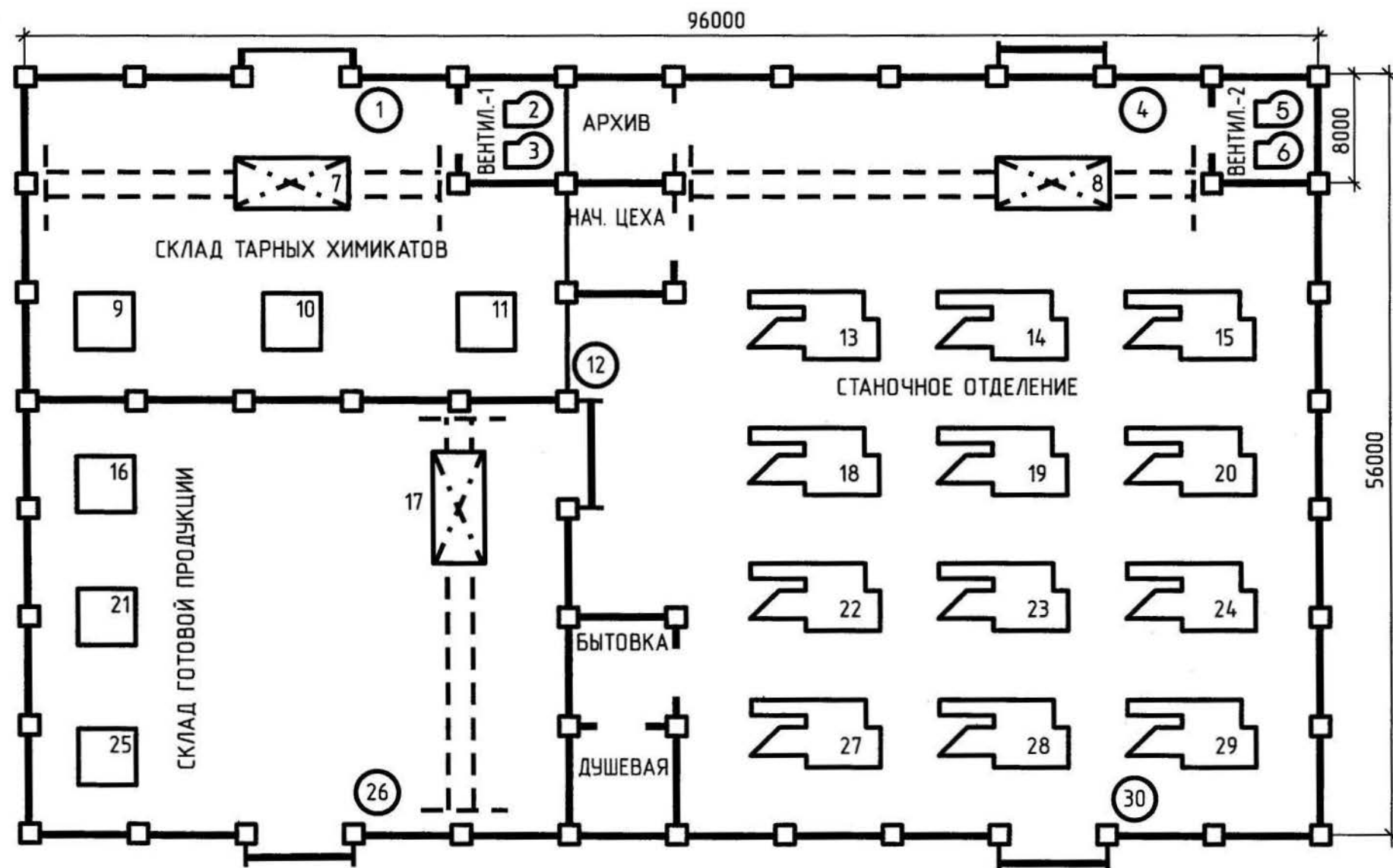
Рис. 3.24. План расположения ЭО шлифовального цеха
