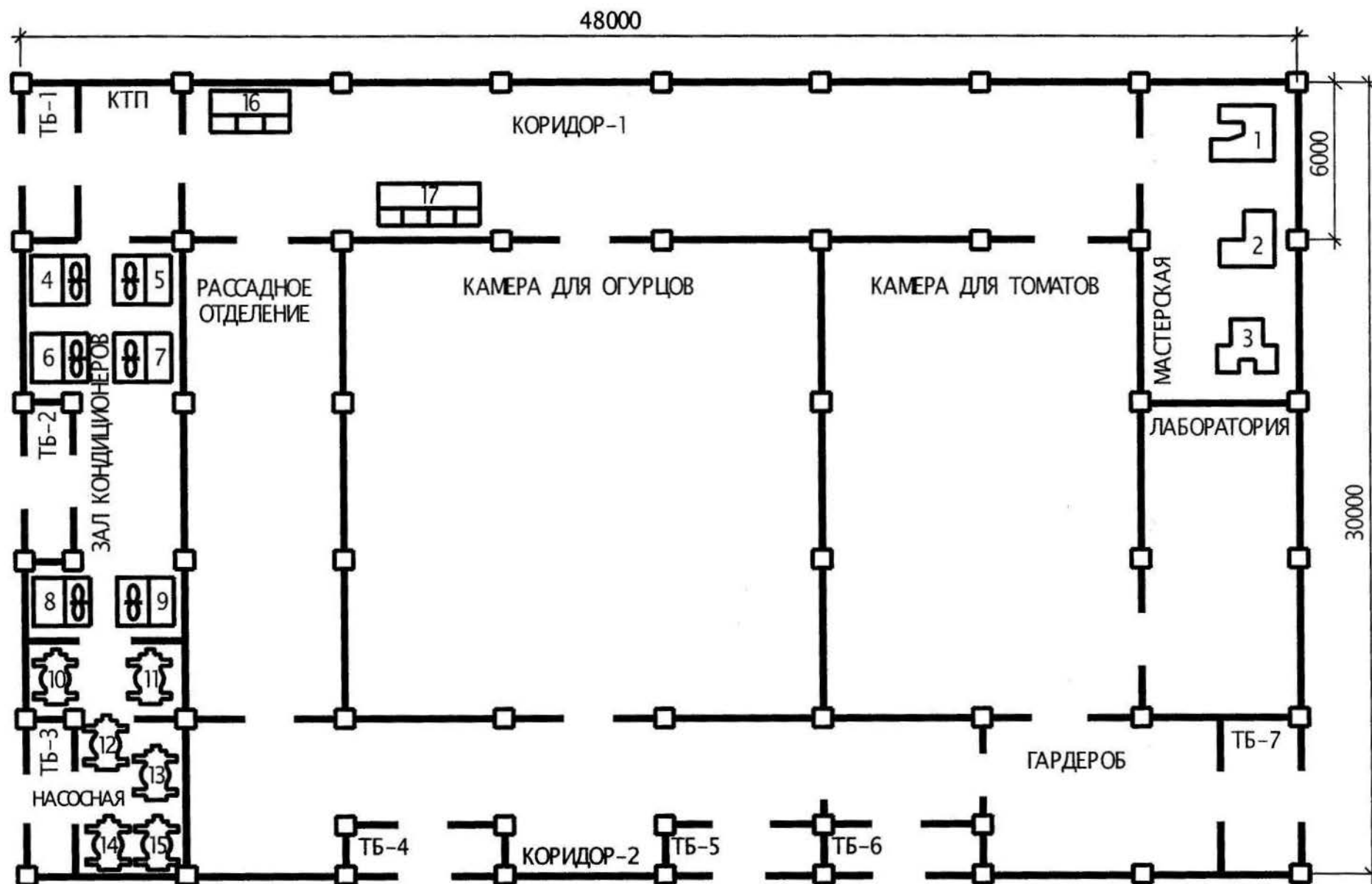
Рис. 3.26. План расположения ЭО светонепроницаемой теплицы
