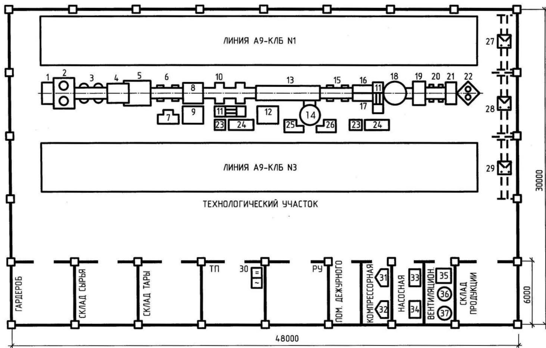
Рис. 3.25. План расположения ЭО комплекса овощных закусовых консервов
