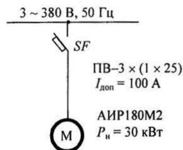
Рис. 1.8.12. Схема линии ЭСН
