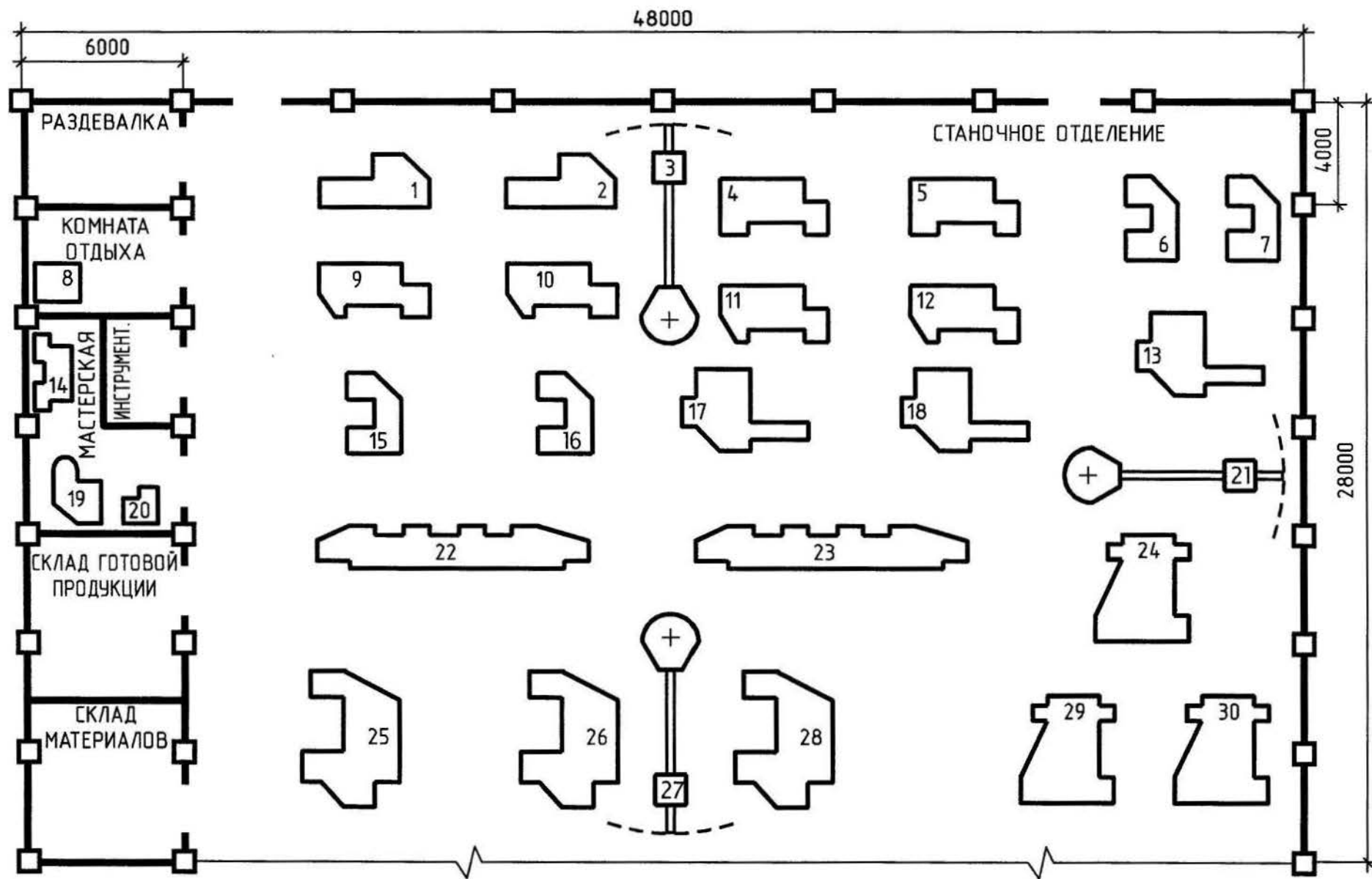
Рис. 3.18. План расположения ЭО участка токарного цеха
