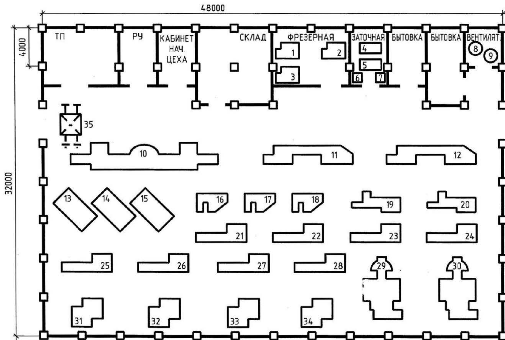
Рис. 3.7. План расположения ЭО механического цеха серийного производства
