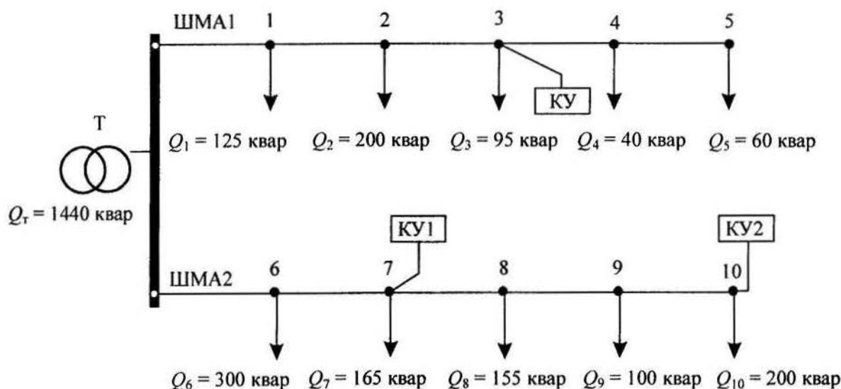
Рис. 1.6.1. Расчетная схема
