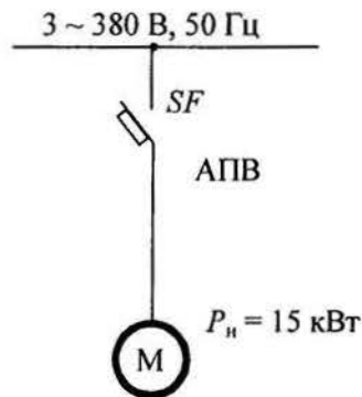
Рис. 1.8.7. Схема линии ЭСН
