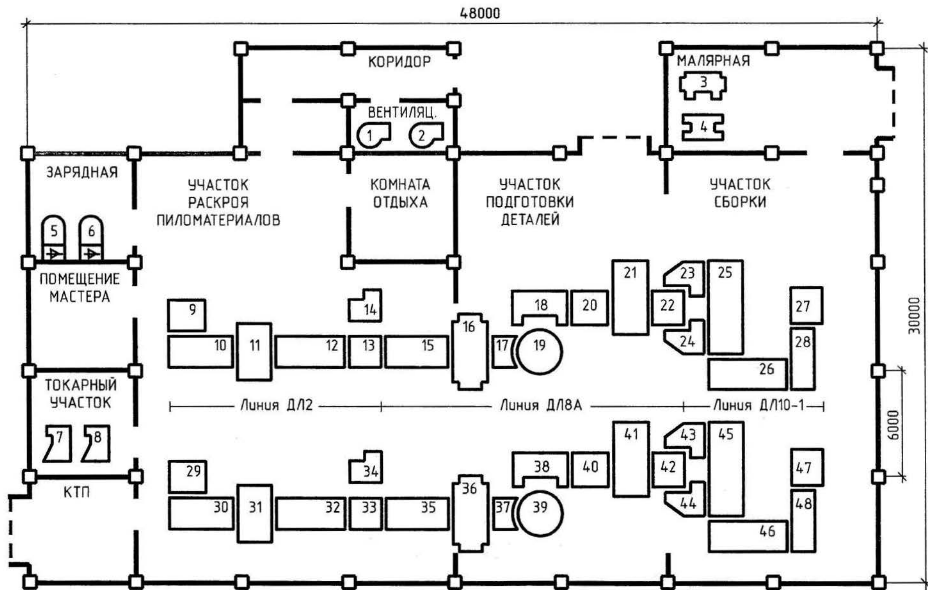
Рис. 3.23. План расположения ЭО деревообрабатывающего цеха
