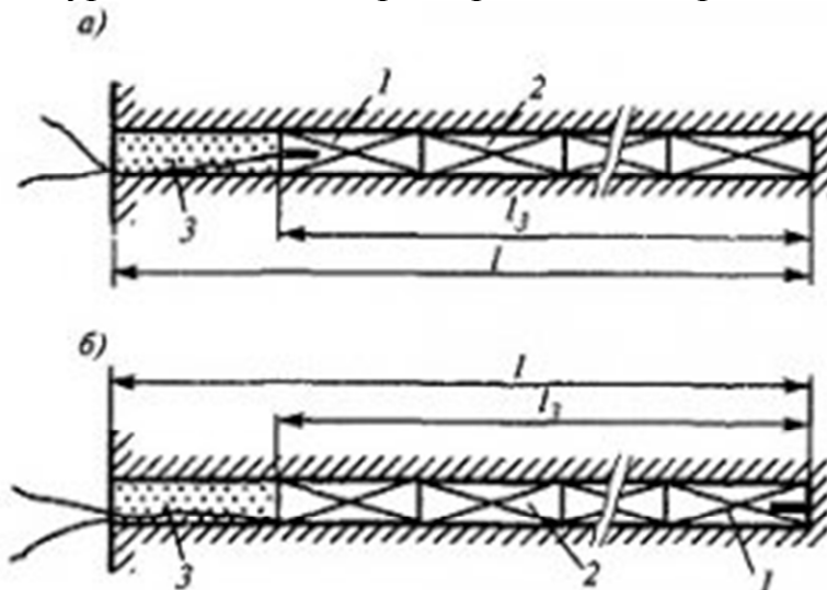
Рис. 9.19. Конструкции сплошных зарядов:
