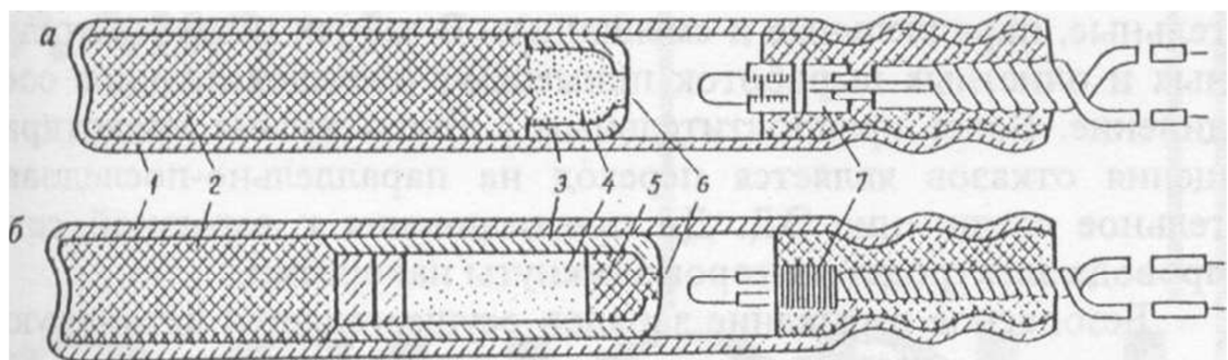
Рис. 3. Электродетонаторы мгновенного (я) и короткозамедленного действия (5): 1 — гильза; 2 — заряд выокобризантиого ВВ; 3 — колпачок-замедлитель; 4 — заряд инициирующего ВВ; 5 — замедляющий состав; 6 — шелковая сеточка; 7 — электровоспламенитель
