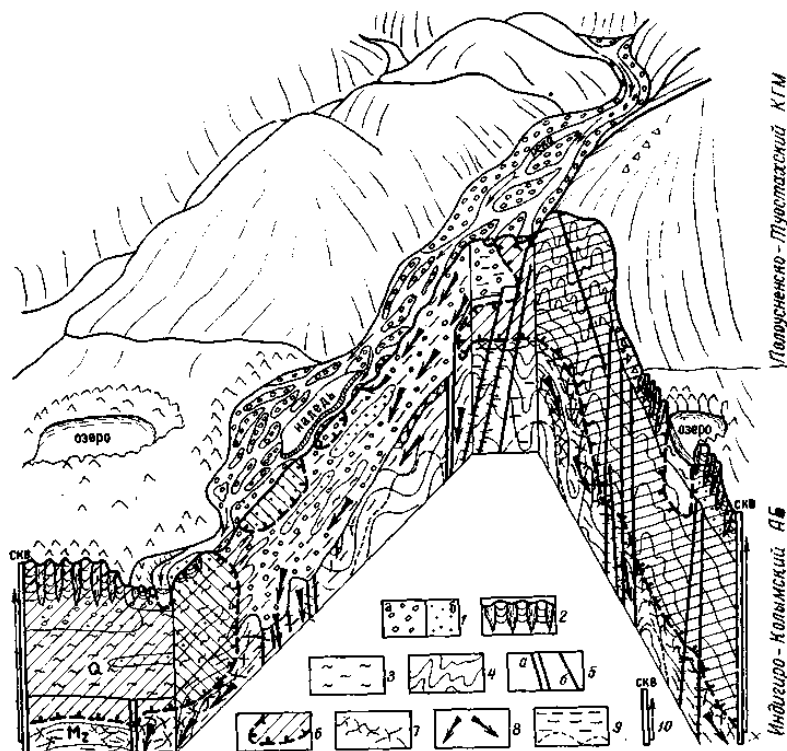
Рис. 2. Схема перелива аллювиальных вод подрусловых и пойменных несквозных таликов из Полуосненского-Туосташского КГМ в Индиго-Колымский АБ глубокого промерзания через сквозной инф<ильтративный талик: / — аллювиальные галечники (а) и пески (б), 2 — аллювиальные пойменные отложения с сингенетическими повторно-жильными льдами, 3 — озерно-аллювиальные суглинки и супеси, 4 — терригенные отложения верхнего мезозоя, в пределах КГМ сложно дислоцированные, 5 — разломы омоложенные (а) и древние (б), 6 — ММП и их граница, 7 — зоны криогенной
