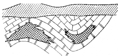
Рис. 7 Линзовидная залежь плавикового шпата в известняках
