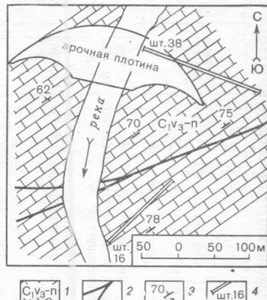
Рис. 1.1. Схематическая геологическая карта долины участка плотины: 1 — известняки мраморизованные, нижнекаменноугольные; 2 — тектонические разломы; 3 — элементы залегания пород; 4 — штольня и ее номер
