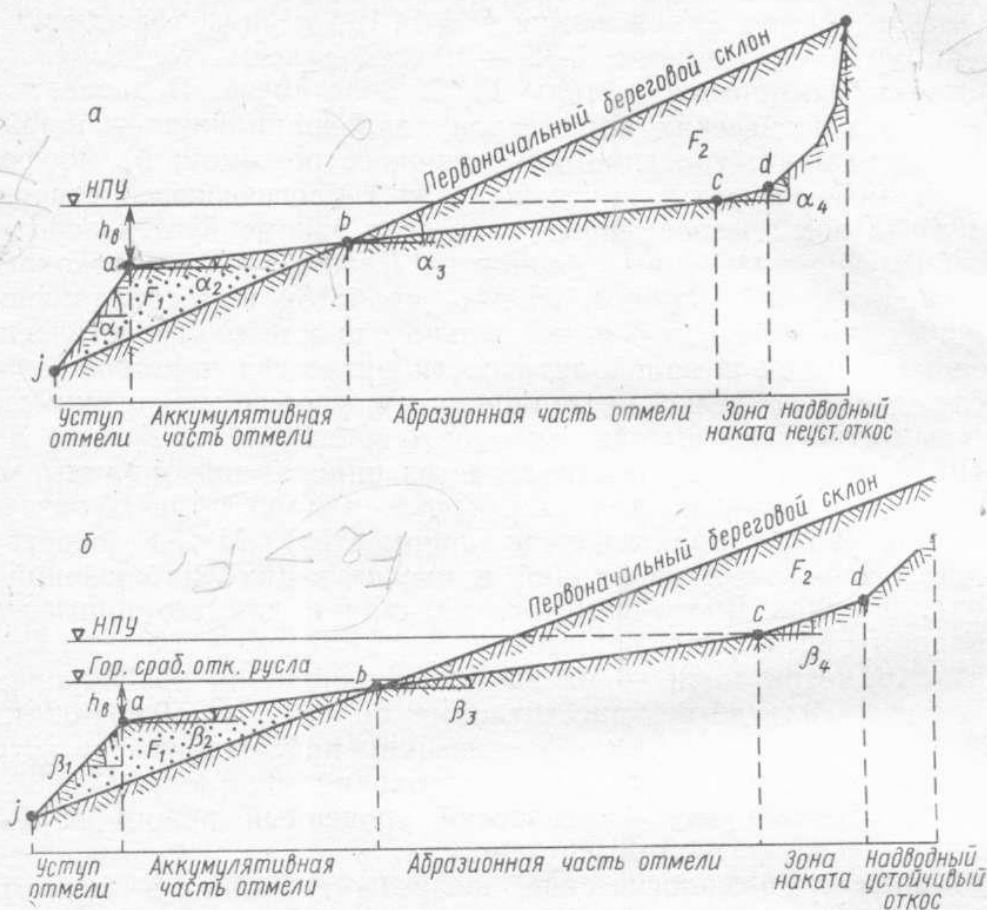
Рис. 6.11. Схема построения береговых отмелей в широкой глубоководной части водохранилища: а — для первой стадии — через 10 лет; б — для конечной стадии практической значимости
