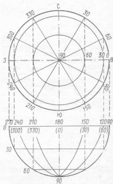
Рис. 6.4. Схема построения полярной сетки
