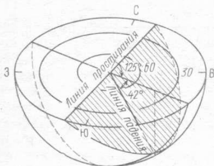
Рис. 6.5. Схема нанесения трещин на полярную сетку. Точка на горизонтальной плоскости соответствует трещине с аз. пад. 125° и \angle 42^\circ . Плоскость трещины заштрихована
