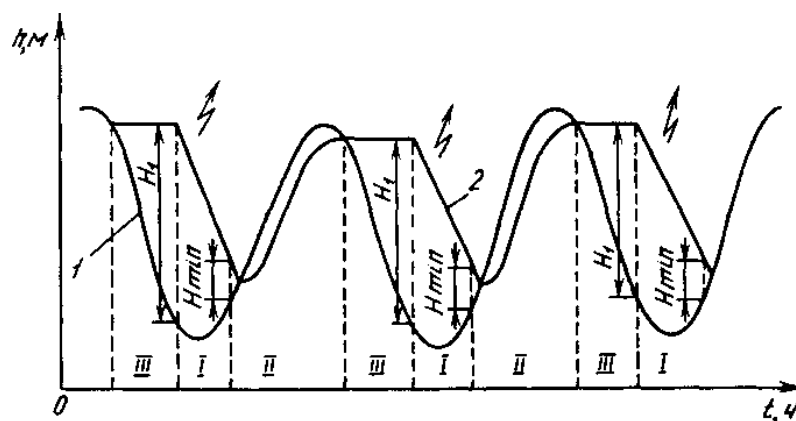
Рис.3. Схема работы однобассейновой ПЭС одностороннего действия:
