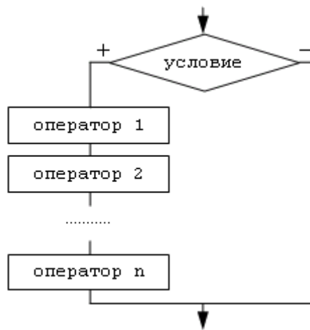
Рисунок 3.8. Неполная форма составного оператора
