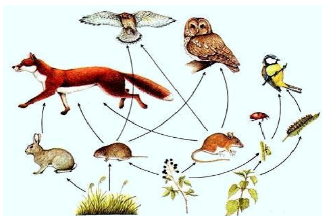
Рисунок 2. Трофическая сеть.
