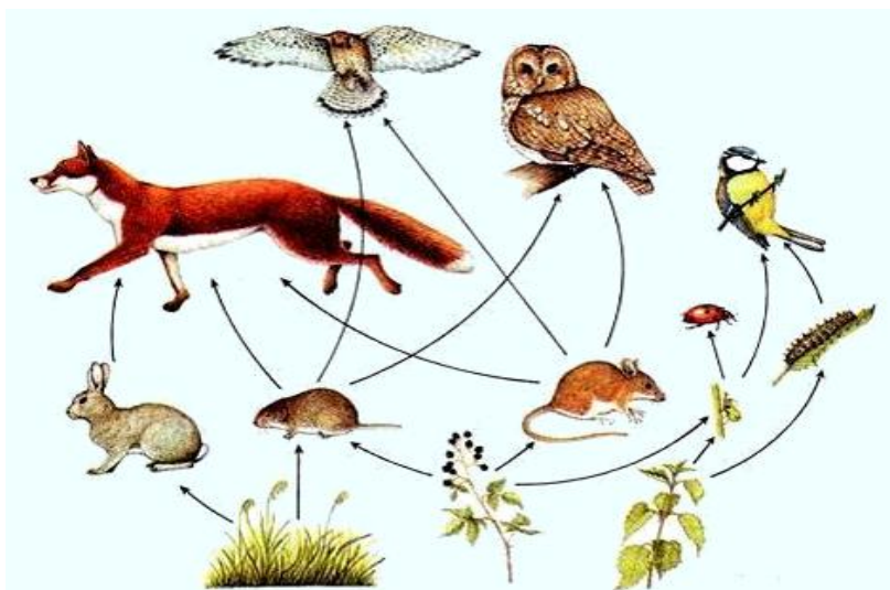
Рисунок 2. Трофическая сеть.
